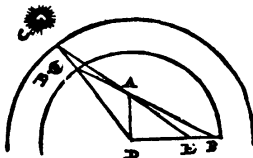
Figura vmbra Luna, Solisq; ostēdens.
