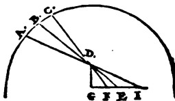
Figura varias Solis vmbra designans.
