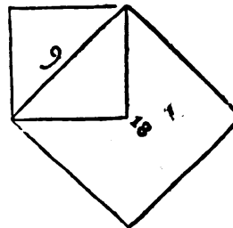
M Figura octo- drati ex diametro quadrati procedit, al- li dupli- catis.
